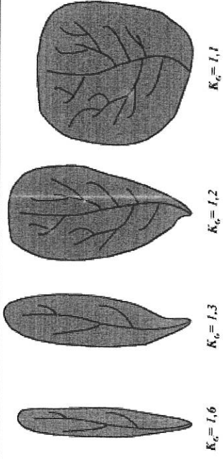
Fig. 2.8 - Exemples d'indices de compacité
