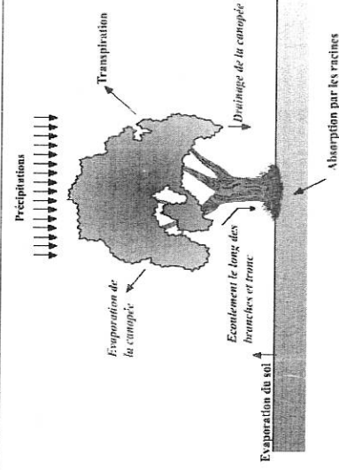
Fig. 4.1 - Principaux éléments intervenant dans les concepts d'interception et d'évapotranspiration.
