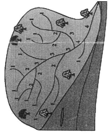
Fig. 2.10 - Classification du réseau hydrographique selon le système de Strahler (1957).
